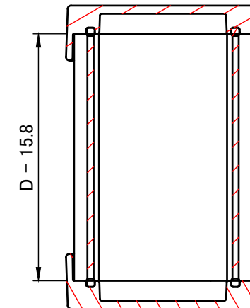
C-C ( 1 : 1.5 )
